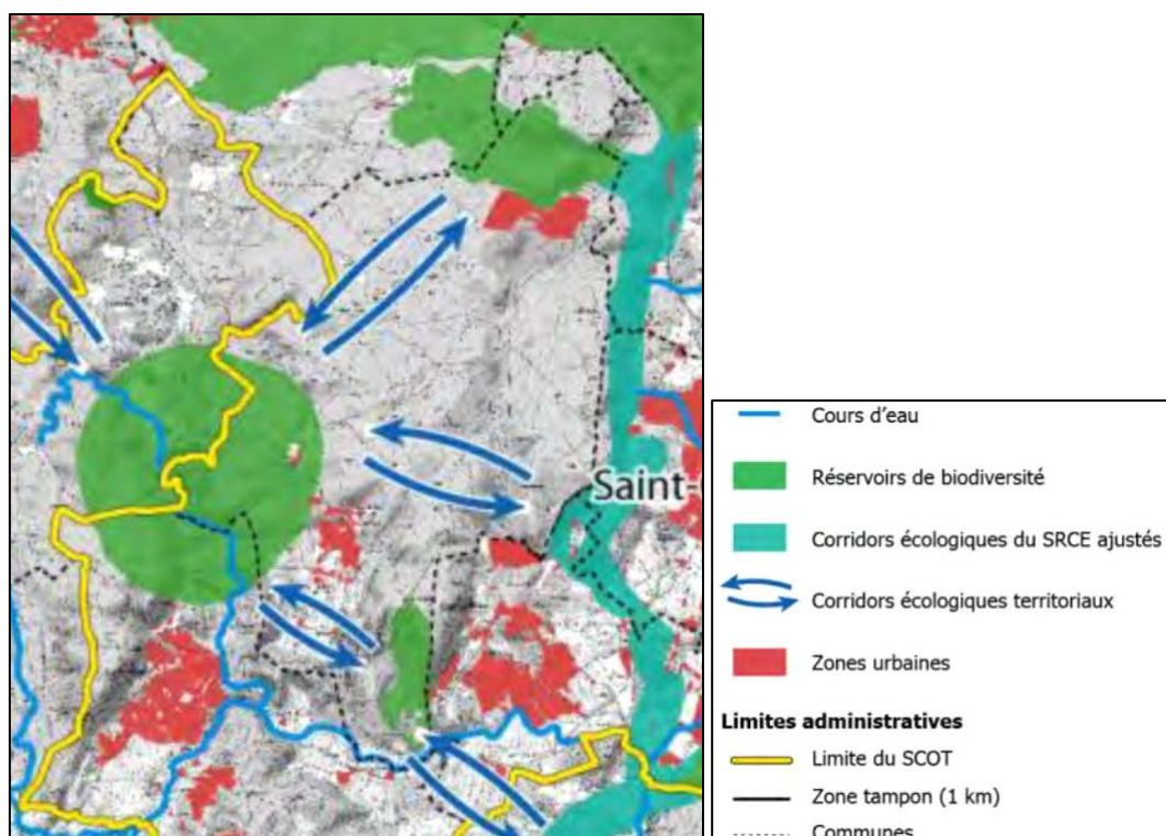
Figure 10 : TVB du SCoT GPSL
