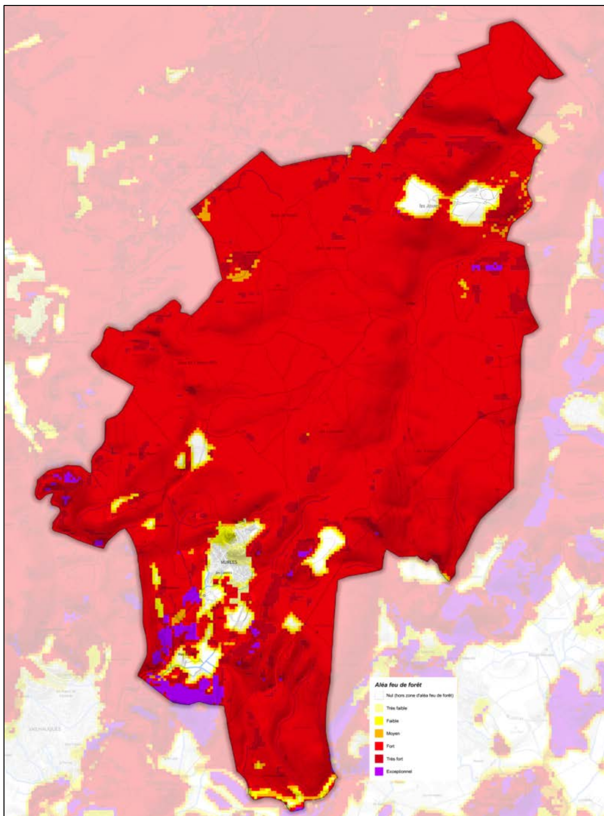
Figure 21 : aléa feu de forêt à l'échelle communale
