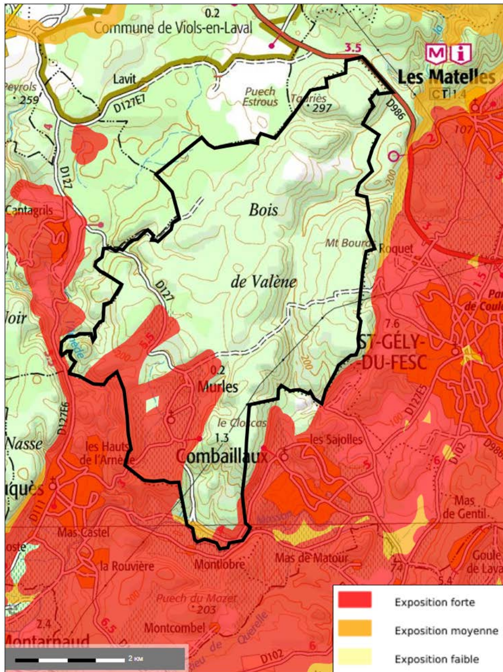
Figure 23 : Exposition au phénomène de retrait-gonflement des argiles
