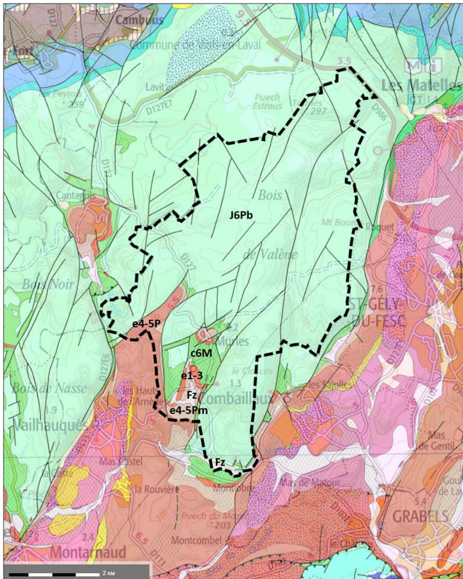
Figure 3 : contexte géologique
